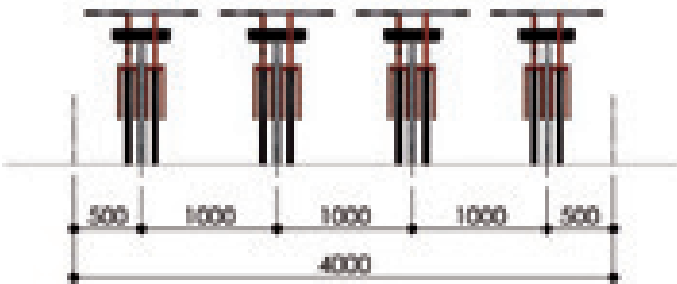
Absperrbügel Achse: 1000 8 Radeinstellungen
