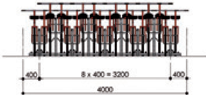
Abspernbügel Achse: 1000 8 Rodeinstellungen
