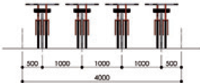
Abspernbügel Achse: 1000 8 Rodeinstellungen
